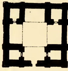
Fig. 108 — Pianta di un sepolcro romano a Kusr en Nubejis nella Palestina
